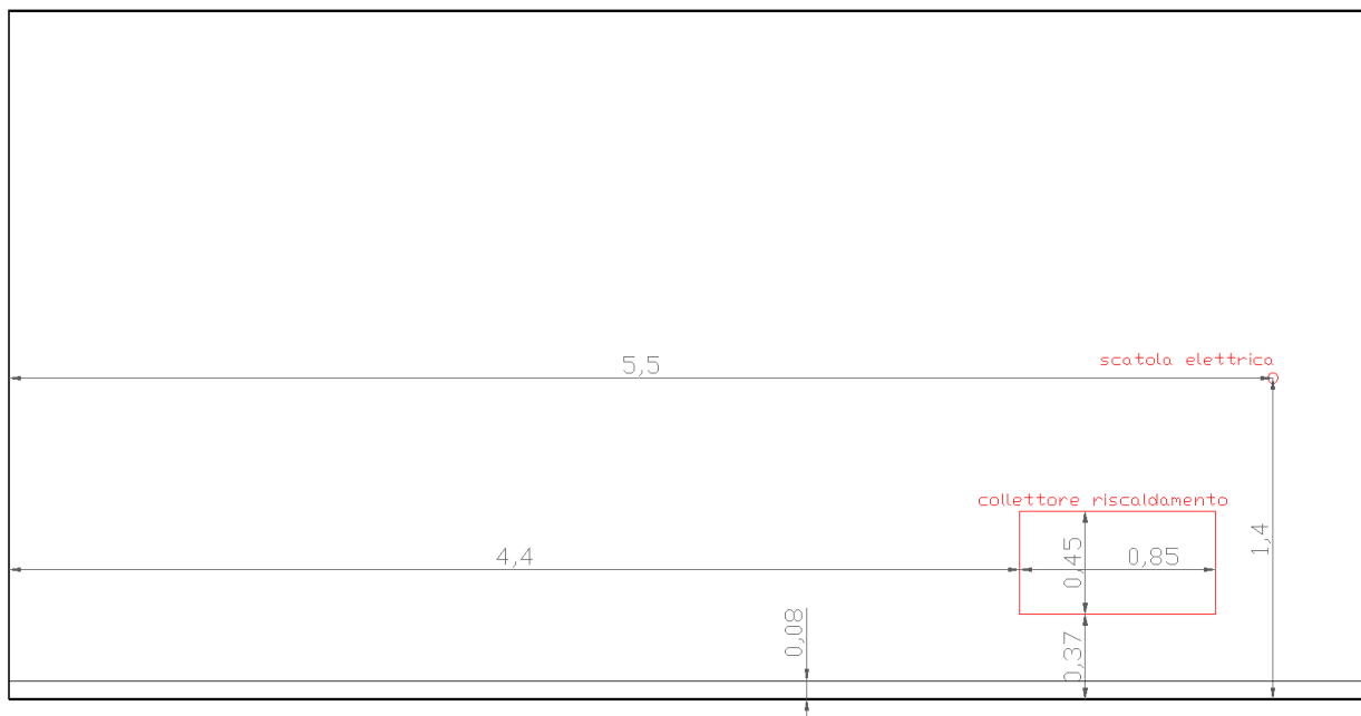
Prospetto della parete con misure
